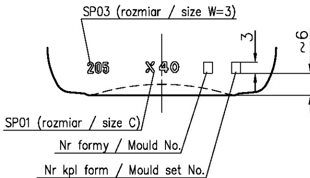
Widok z przodu / Front view
